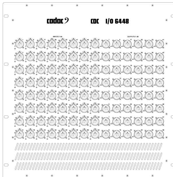
18: CDC I/O 6448 Stagebox
